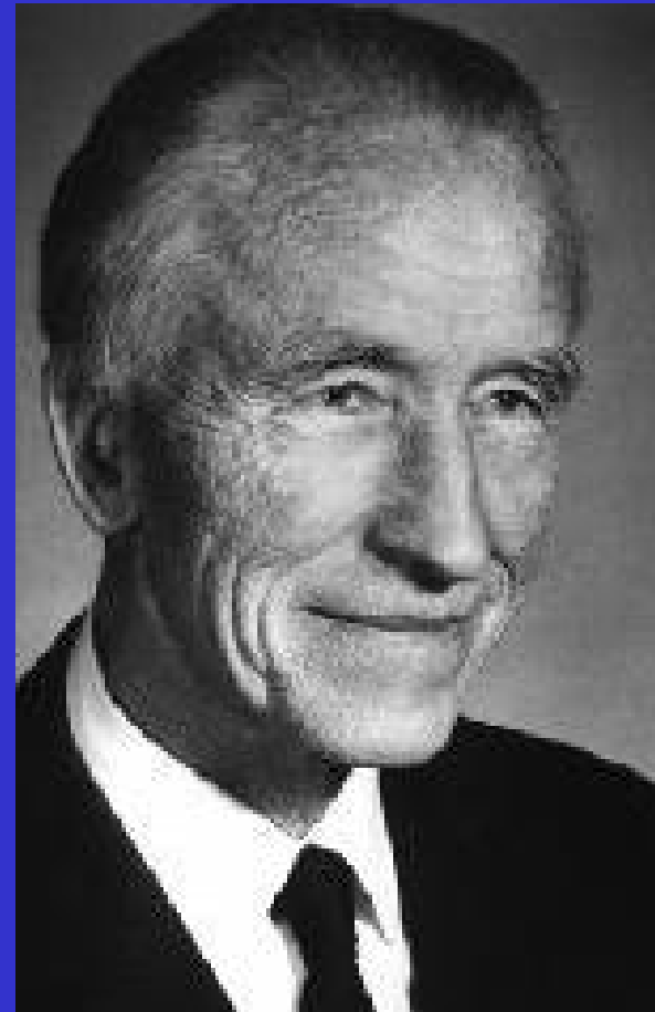
Jacob Bjerknes (1897-1975)
