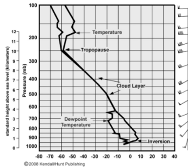
Stuve Diagram
